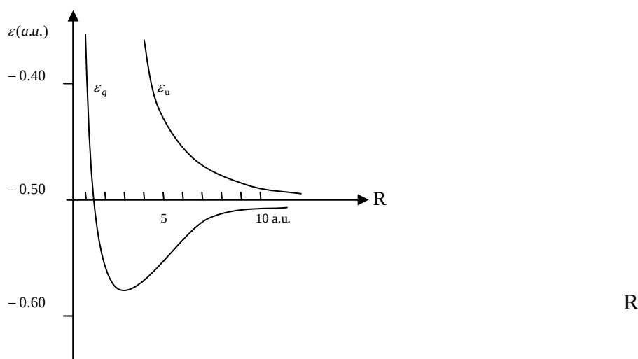
ل (2.2) - انرژی کل یون H_2^+ که تابعی از فاصله بستگی برای در حالت \varphi_g و \varphi_u است رسم شده است.
