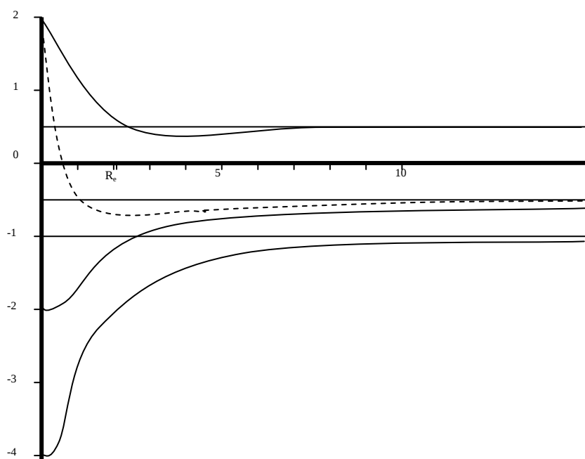
شکل 2.5: انرژی های جنبشی پتانسیل و انرژی الکترون ( \langle \hat{T} \rangle_g, \langle \hat{V} \rangle_g ) و E_g را برای یون H_2^+ بعنوان تابعی از فاصله پیوند R برای تابع موجی که با اوربیتال توانی بهینه سازی شده است را نشان می دهد. منحنی خط چین انرژی کل \epsilon_g و خطوط افقی مقادیر را برای R = \infty نشان می دهند.
